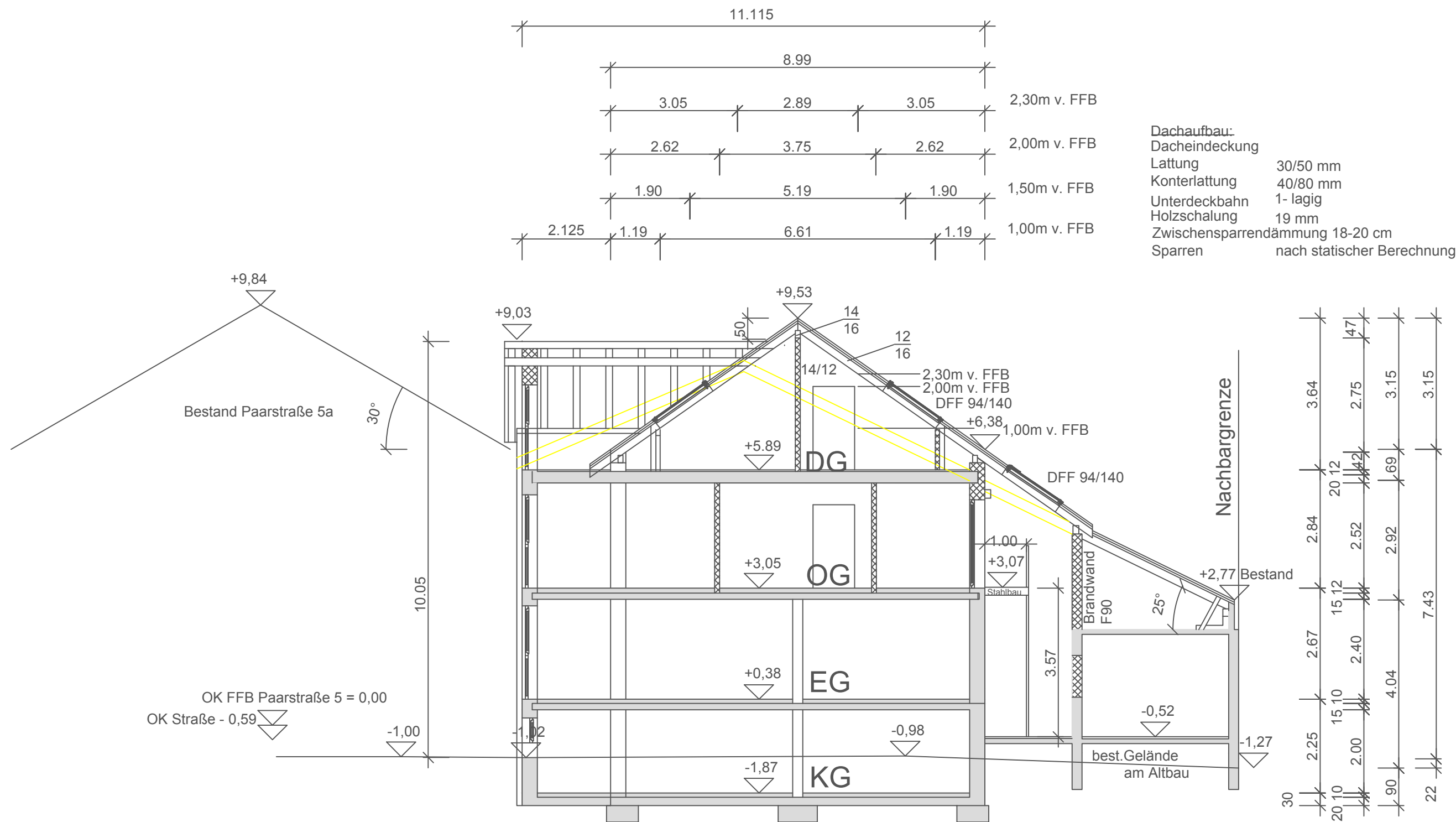
Schnitt Altbau B-B M1:100
